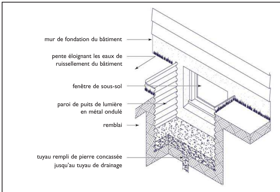
Figure 4 Paroi de puits de lumière contre le mur de fondation
