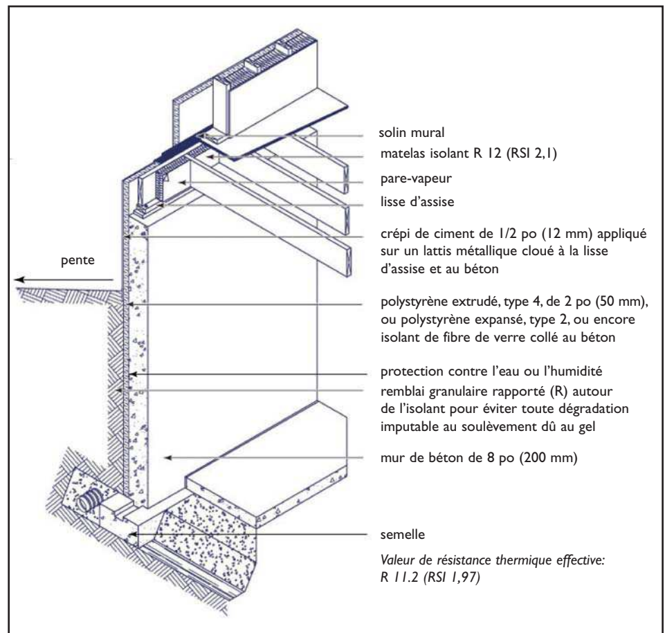
Figure 3 Mur de fondation en béton isolé sur sa face extérieure
